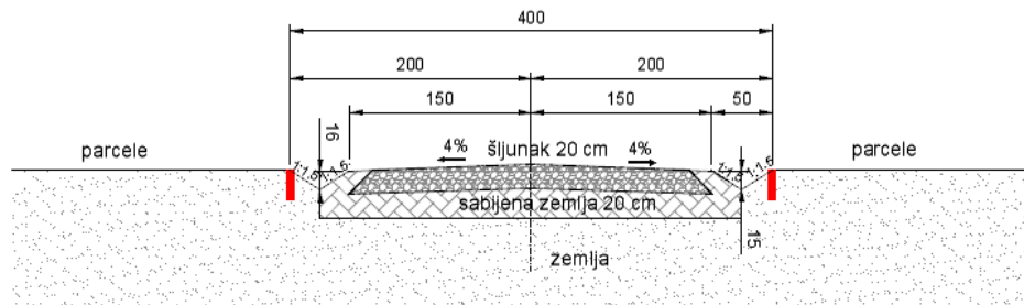
normalni presek 6 - 6
