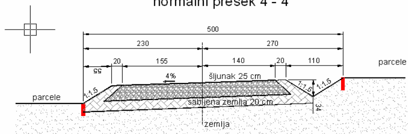
normalni presek 4 - 4
