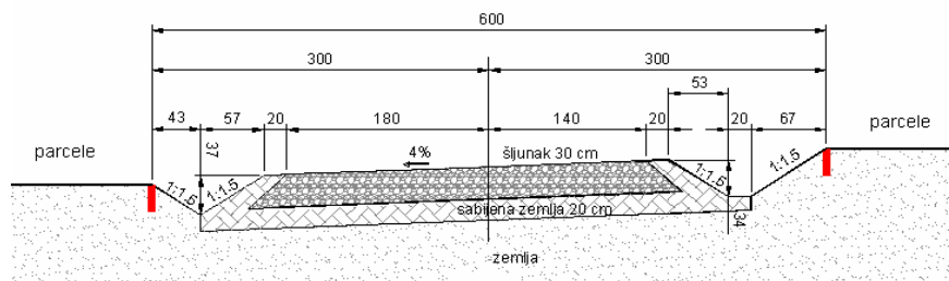
normalni presek 1 - 1
