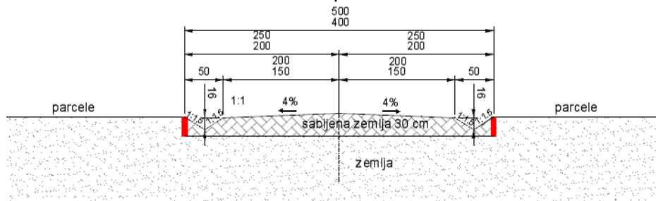
normalni presek 7 - 7
