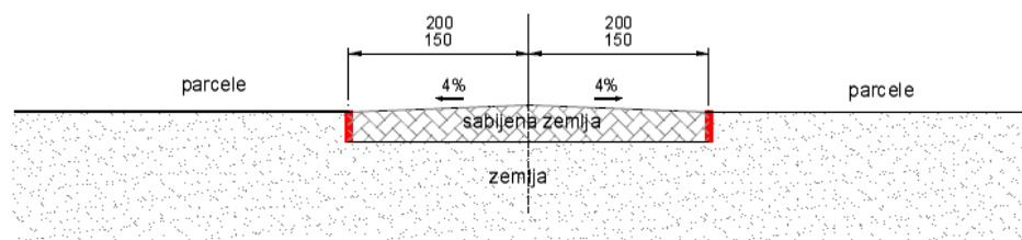
normalni presek 8 - 8
