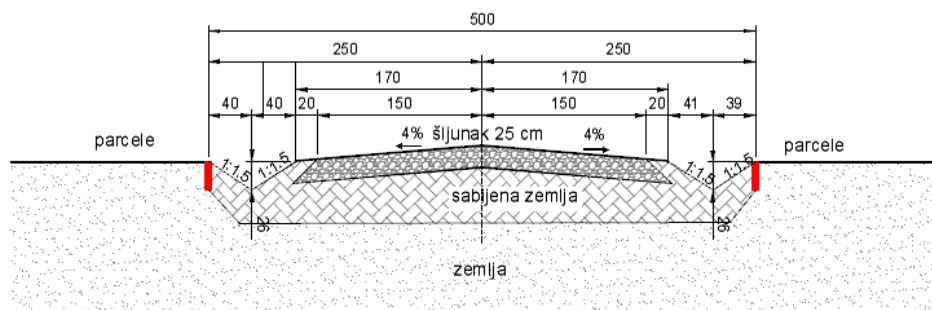
normalni presek 5 - 5
