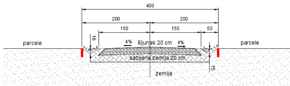
normalni presek 6 - 6
