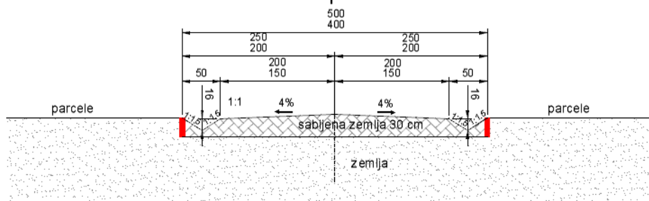
normalni presek 7 - 7
