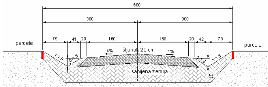
normalni presek 3 -3
