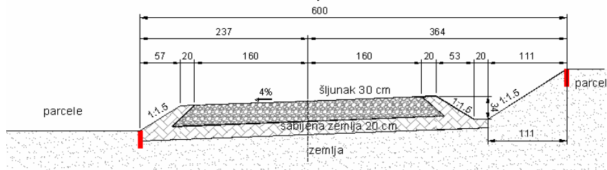
normalni presek 2 - 2
