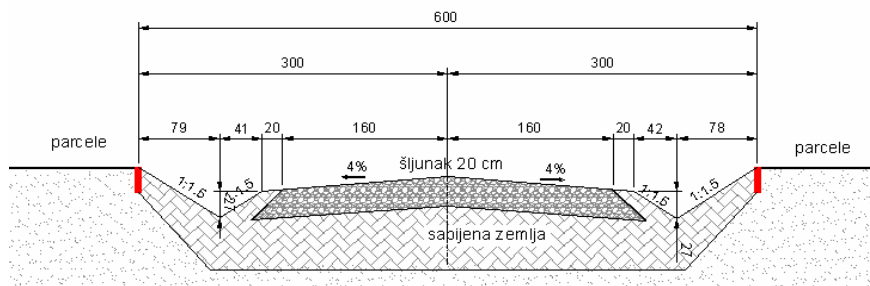
normalni presek 3 -3
