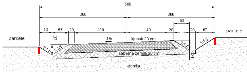
normalni presek 1 -1
