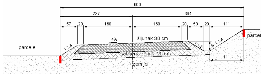
normalni presek 2 - 2
