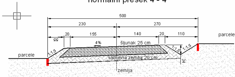
normalni presek 4 - 4
